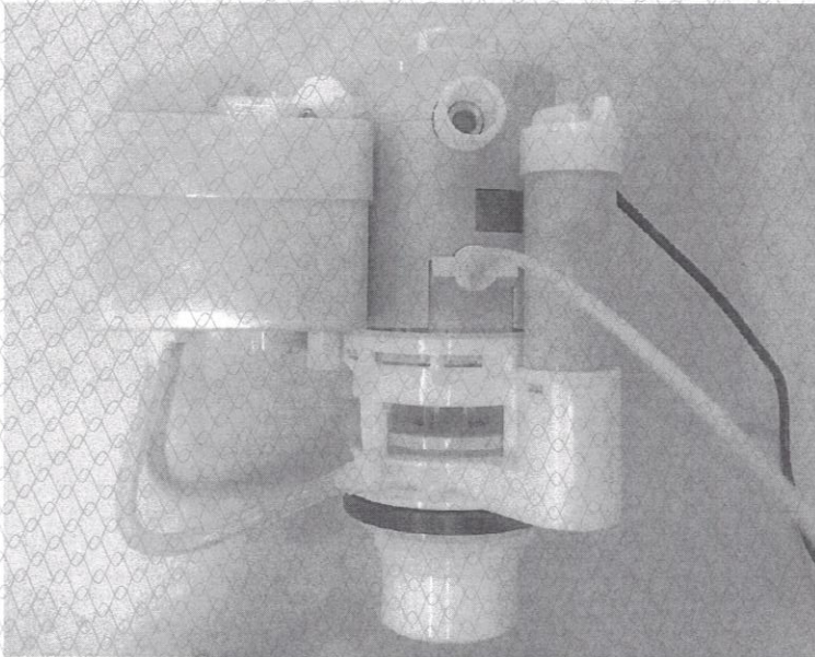
关键零部件照片 (水箱配件或冲洗阀、进水电磁阀)
